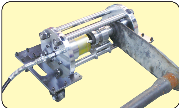
TR-600 series スタビライザーブッシュ交換機
