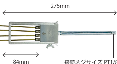
接続ネジサイズ PT1/8
