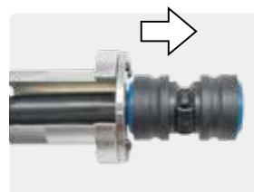
奥の爪を押し、 チューブが抜けます
