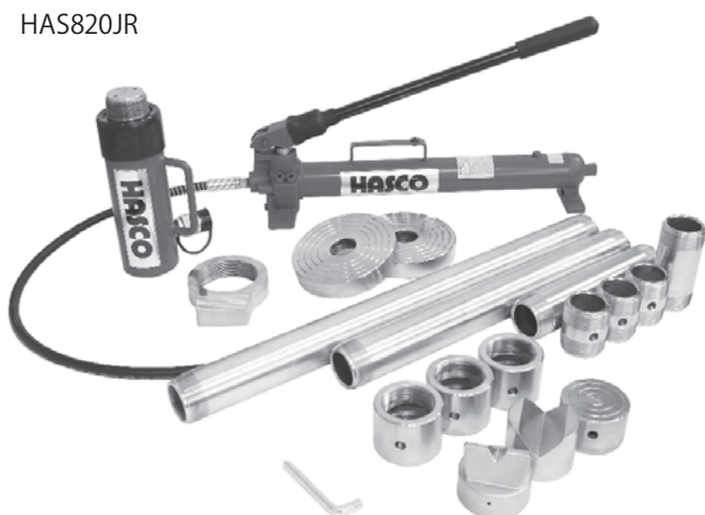
● HAS820JR：油圧ハンドラムセット (20t/19点 set)
