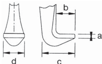
各種爪先端サイズ一覧 (単位: mm)
