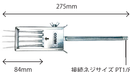
GR-550-02 ノズル (4 本 1 組 / ネジ式)
