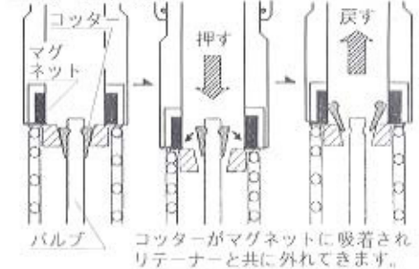
コッター装着の原理
