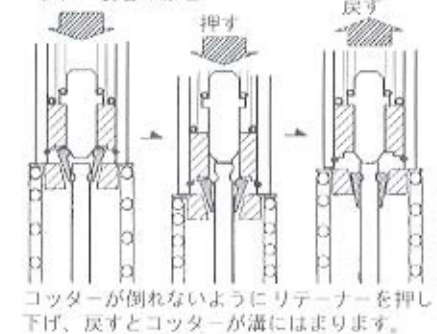
コッター装着の原理
