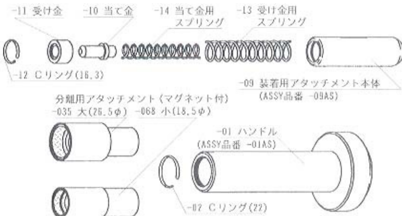
部品展開図・パーツリスト
