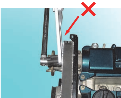
カムプーリーに合う固定ピンを選び 本体及びスイングアームを左右に開く
