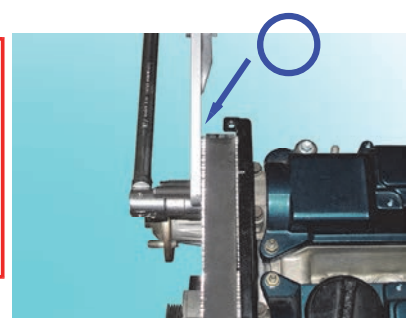
カムプーリーと工具本体がガタが 無いことを確認してから センターボルトをゆるめます。
